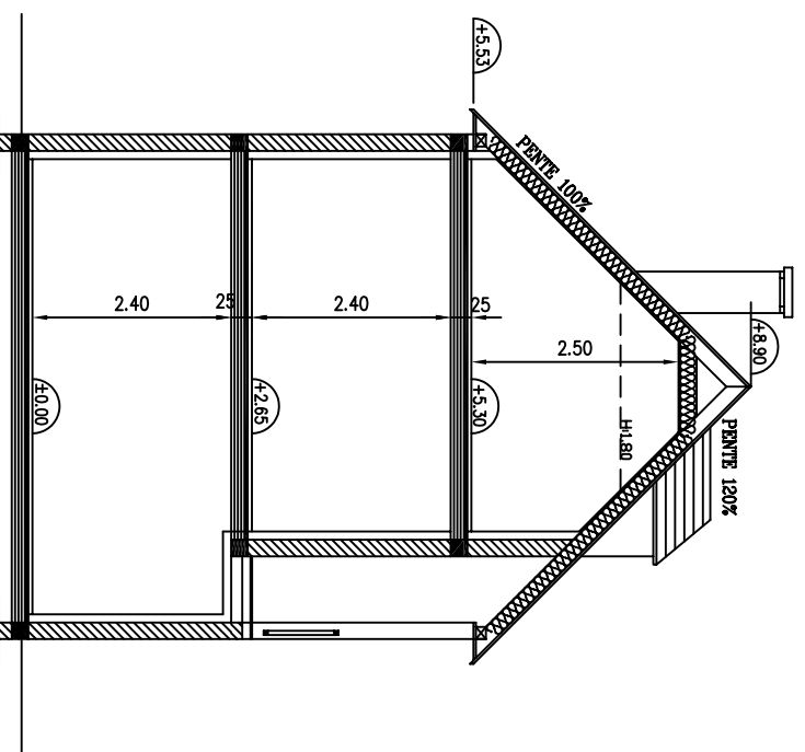
COUPE
