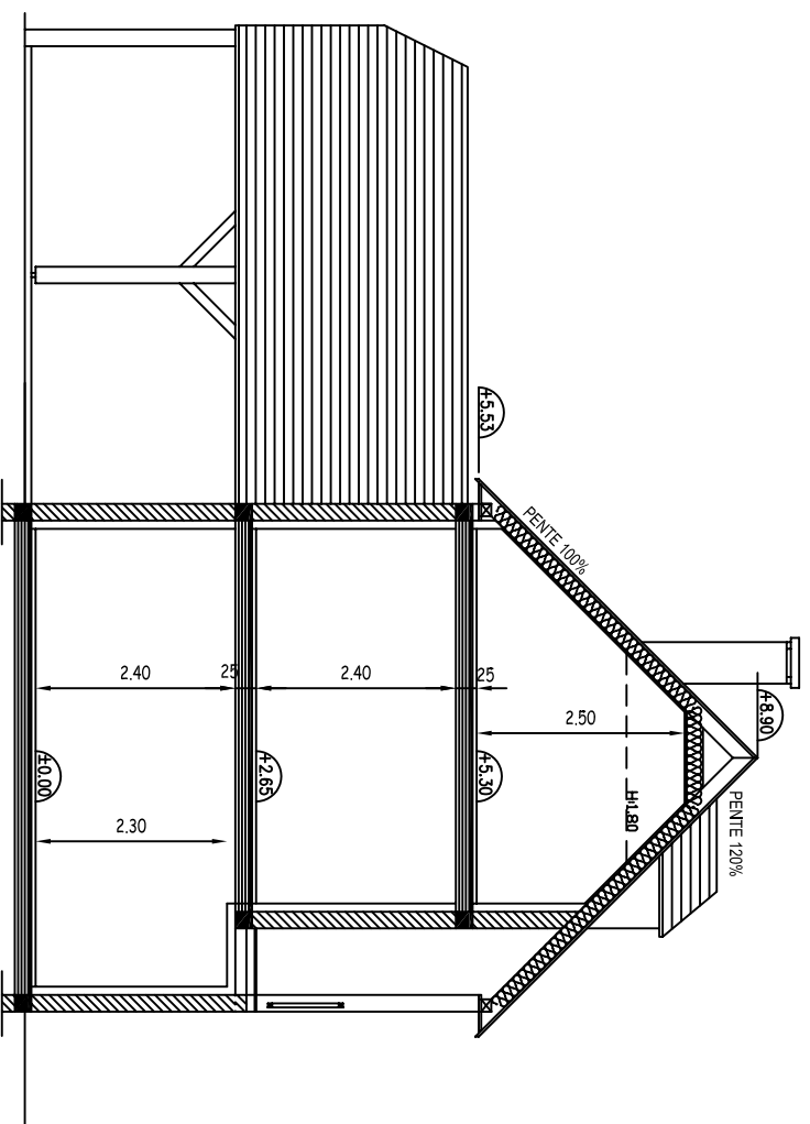
COUPE
