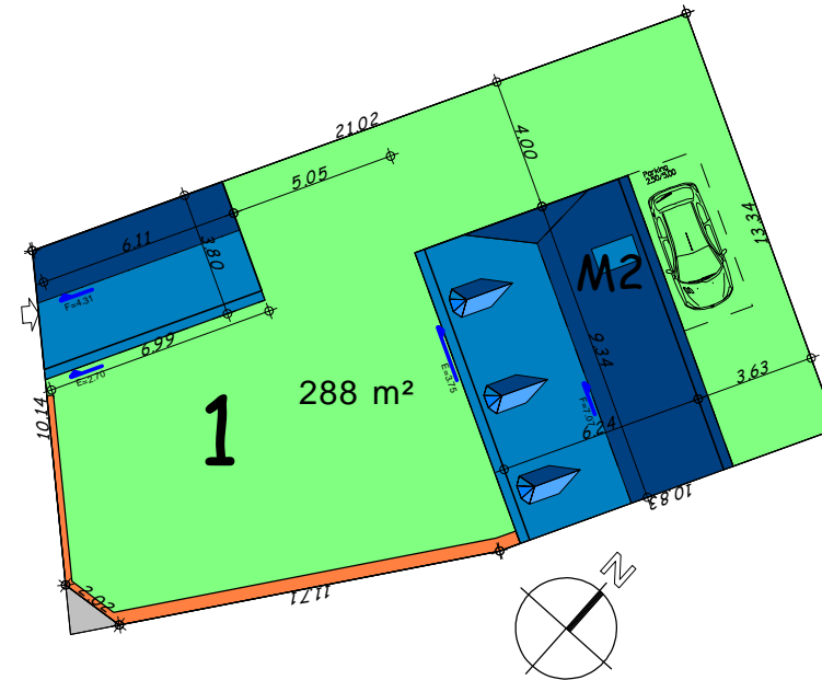
Plan de masse 1/250
