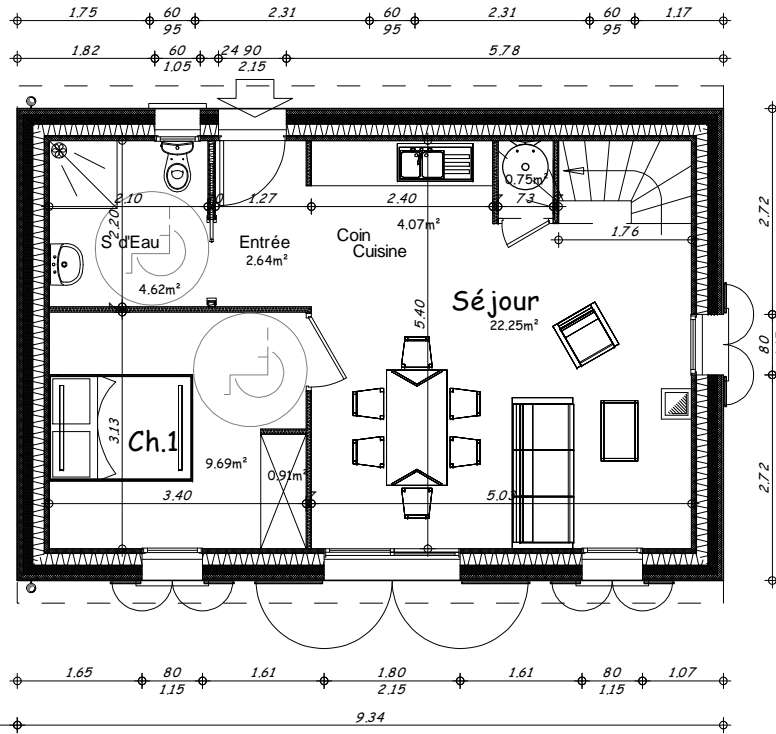
Plan Rez de Chaussée 1/100
