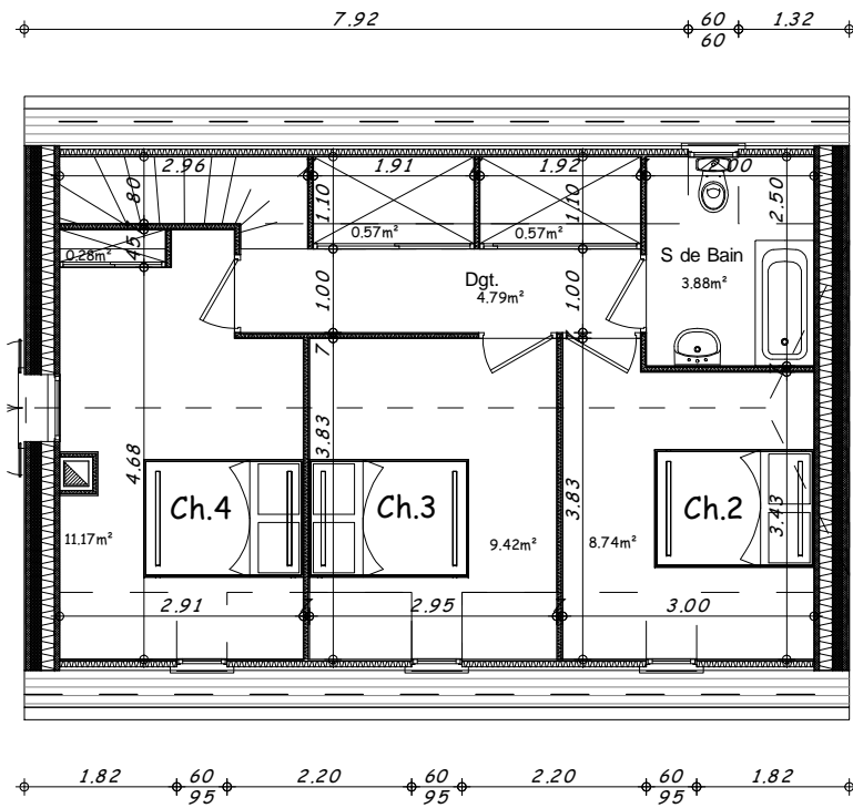
Plan Etage 1/100
