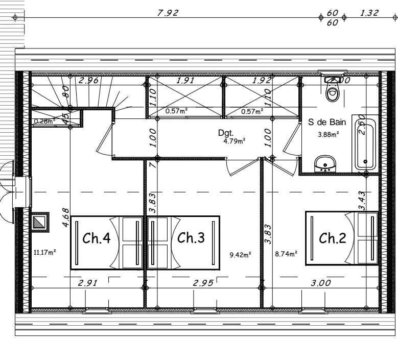
Plan Etage 1/100
