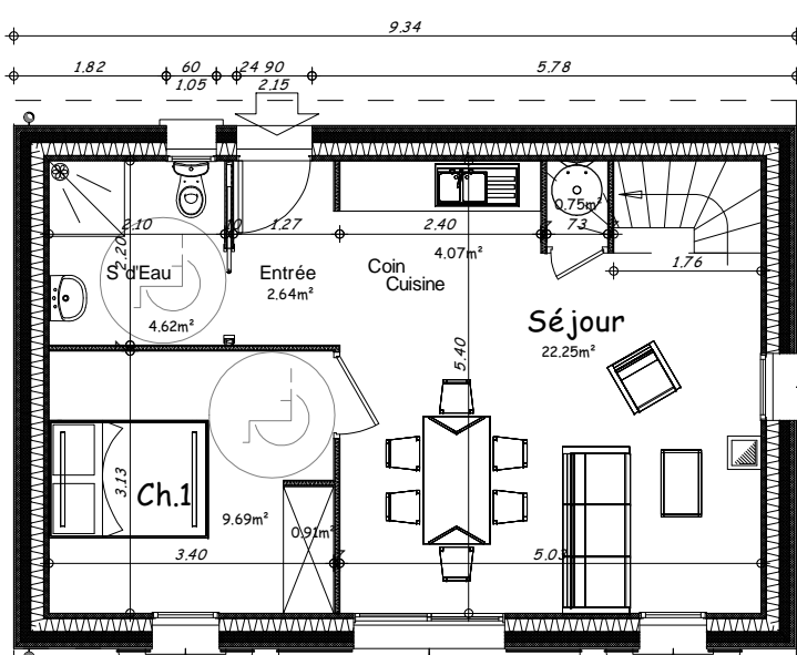
Plan Rez de Chaussée 1/100
