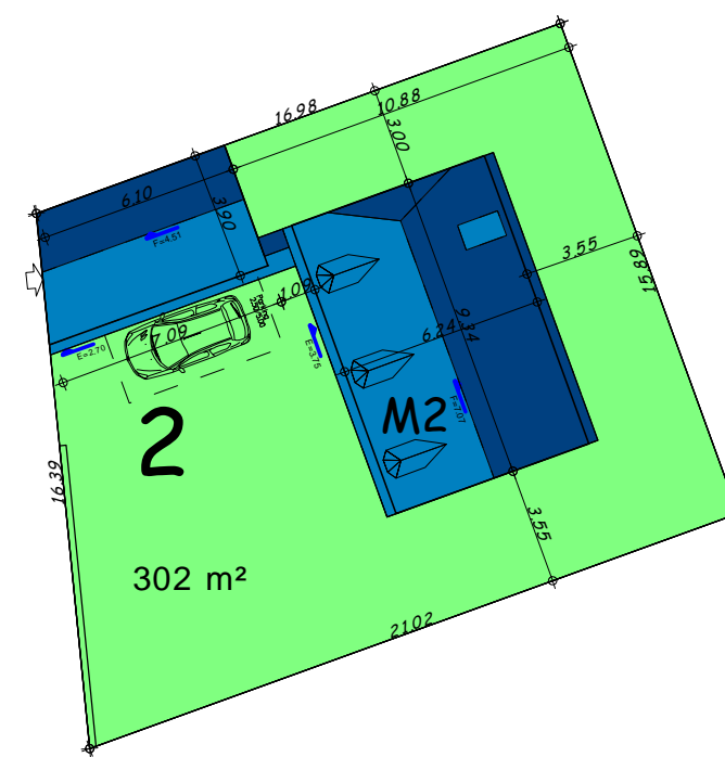
Plan de masse 1/250
