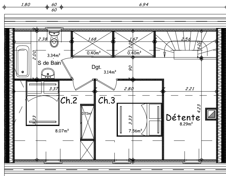
Plan Etage 1/100
