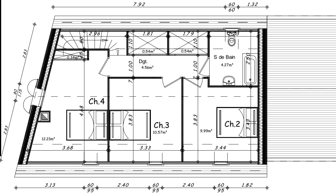
Plan Etage 1/100
