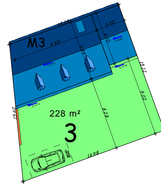
Plan de masse 1/250
