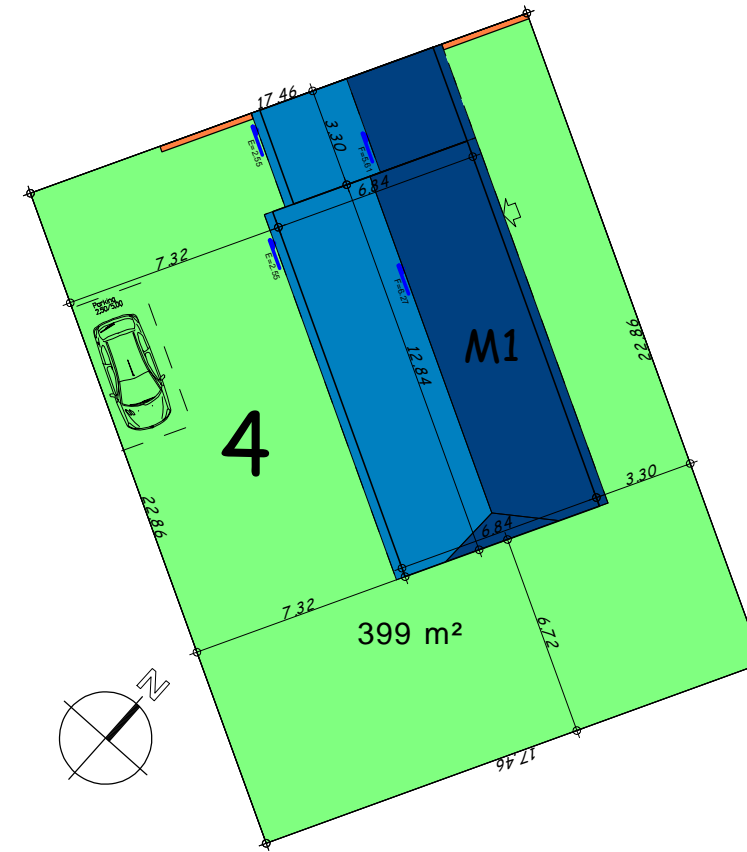
Plan de masse 1/250
