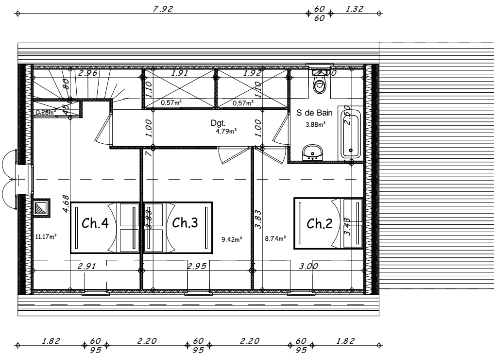
Plan Etage 1/100
