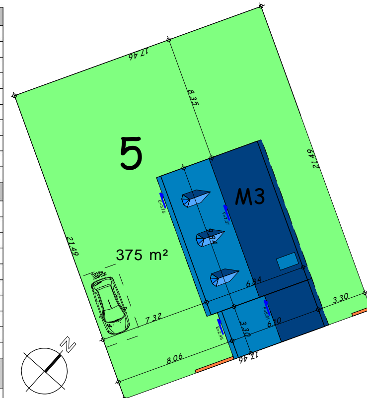
Plan de masse 1/250
