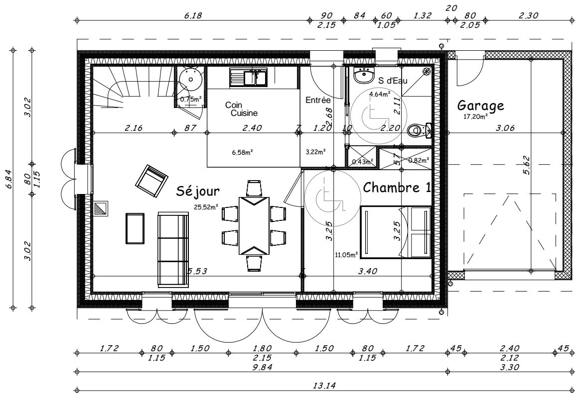
Plan Rez de Chaussée 1/100
