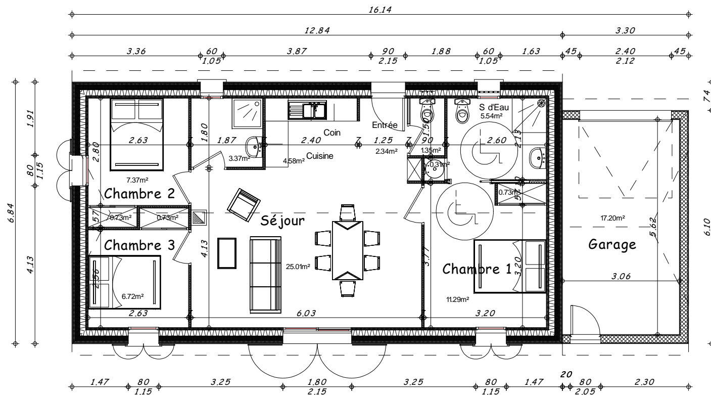
Plan Rez de Chaussée 1/100
