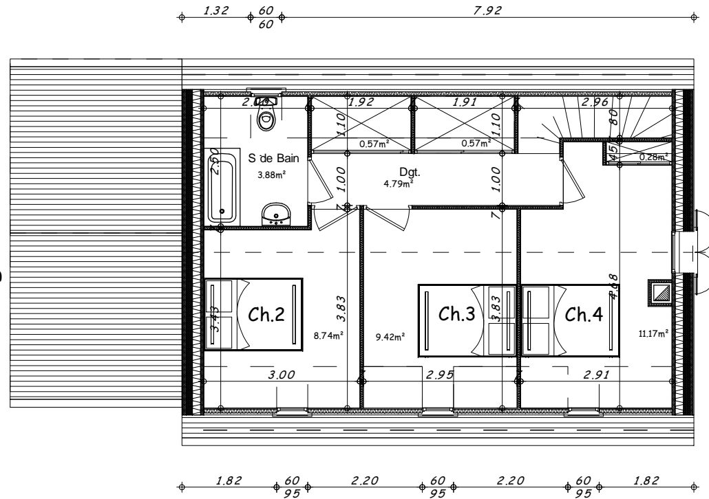
Plan Etage 1/100
