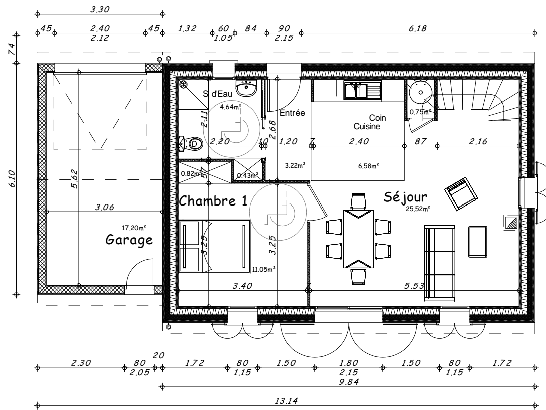
Plan Rez de Chaussée 1/100
